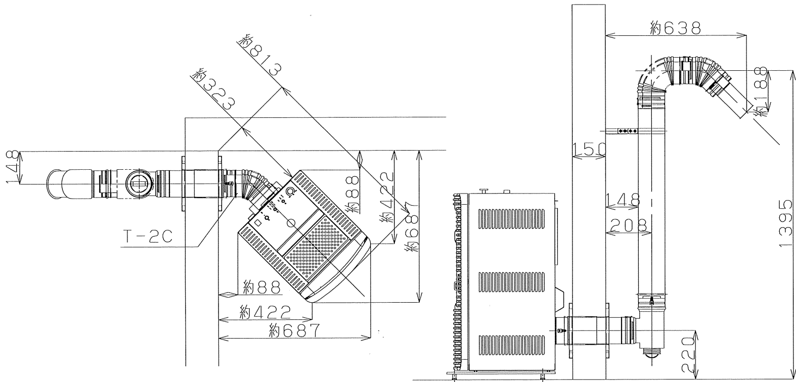
PE-6CT標準設置図
